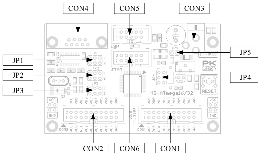
Obr. 2 - rozmístění konektorů a propojek na základové desce
