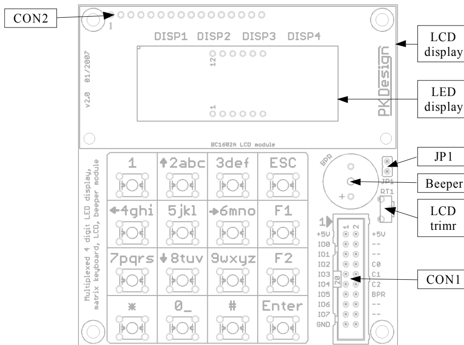
Obr. 1 - umístění konektorů a propojek
