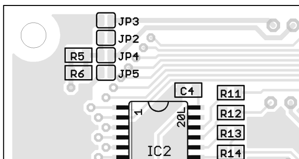
Obr. 3 - umístění propojek na spodní straně desky plošných spojů modulu
